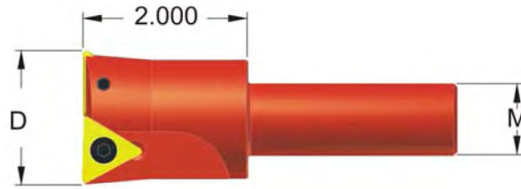
INTERLOC SPOT FACER TOOL
